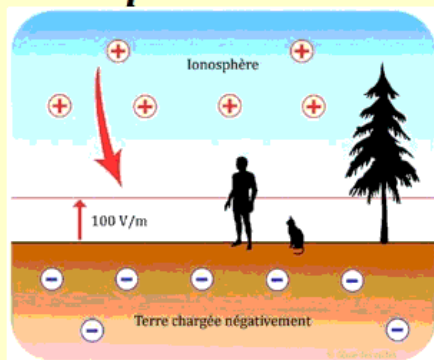
Champ Electrique Terrestre
