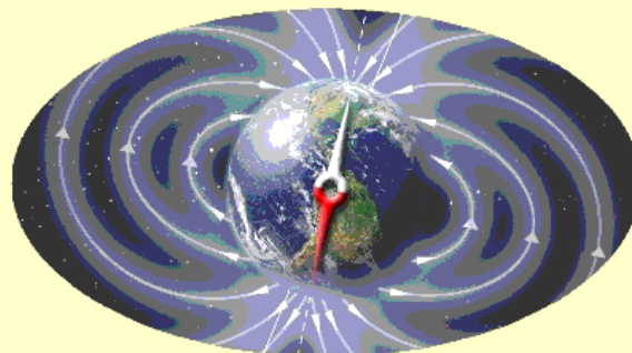
Champ Magnétique Terrestre
