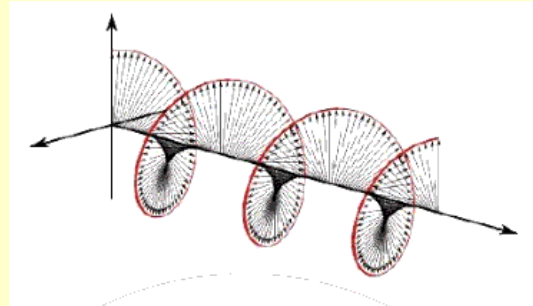
Ondes Scalaires
