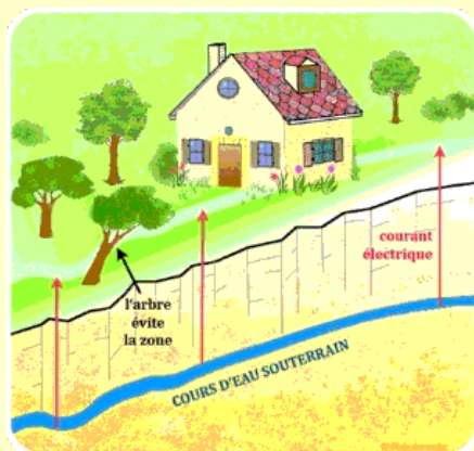
Courant Tellurique (Géobiologie)
